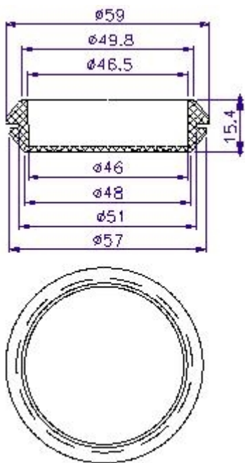
FIGURA 10. TAPON REMOVIBLE - PASACABLES (forma sugerida)
