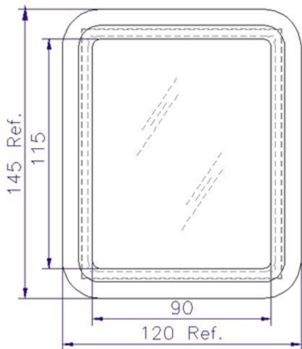
FIGURA 7. VENTANA DE INSPECCION
