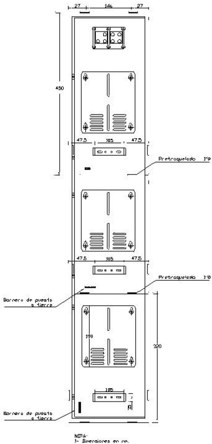
FIGURA 2. VISTA FRONTAL - INTERIOR
