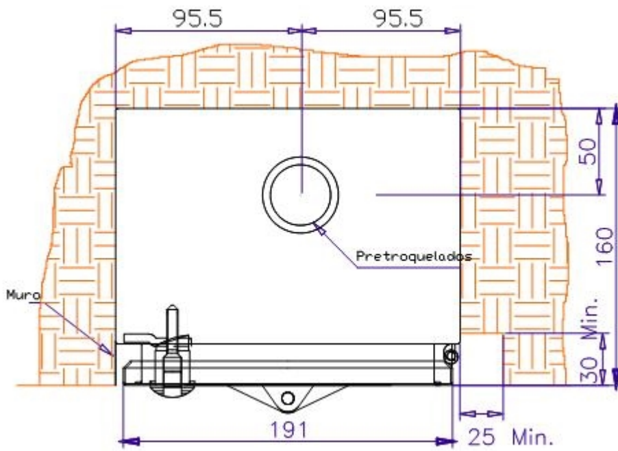
FIGURA 4. VISTA SUPERIOR
