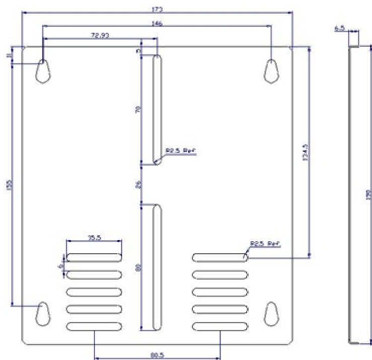
FIGURA 6. BANDEJA PARA MEDIDOR MONOFÁSICO
