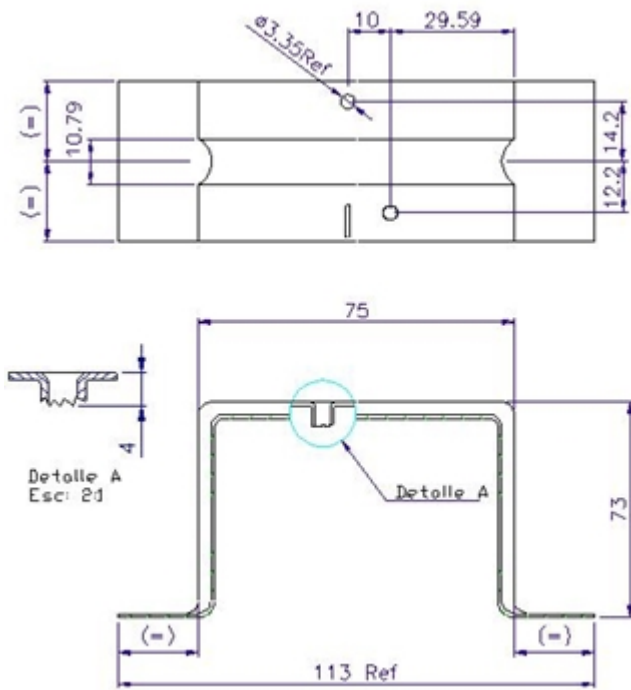
FIGURA 8. SOPORTE INTERRUPTOR
