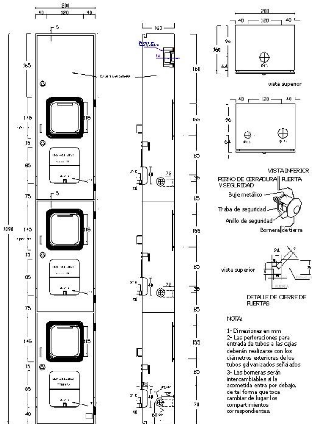
FIGURA 3 VISTA LATERAL
