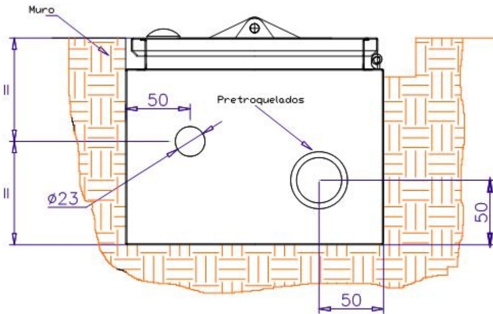
FIGURA 5. VISTA INFERIOR
