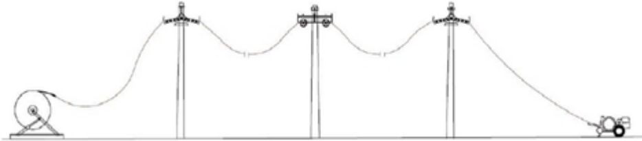
Figura No. 6 Esquema instalación de cable cuádruplex
