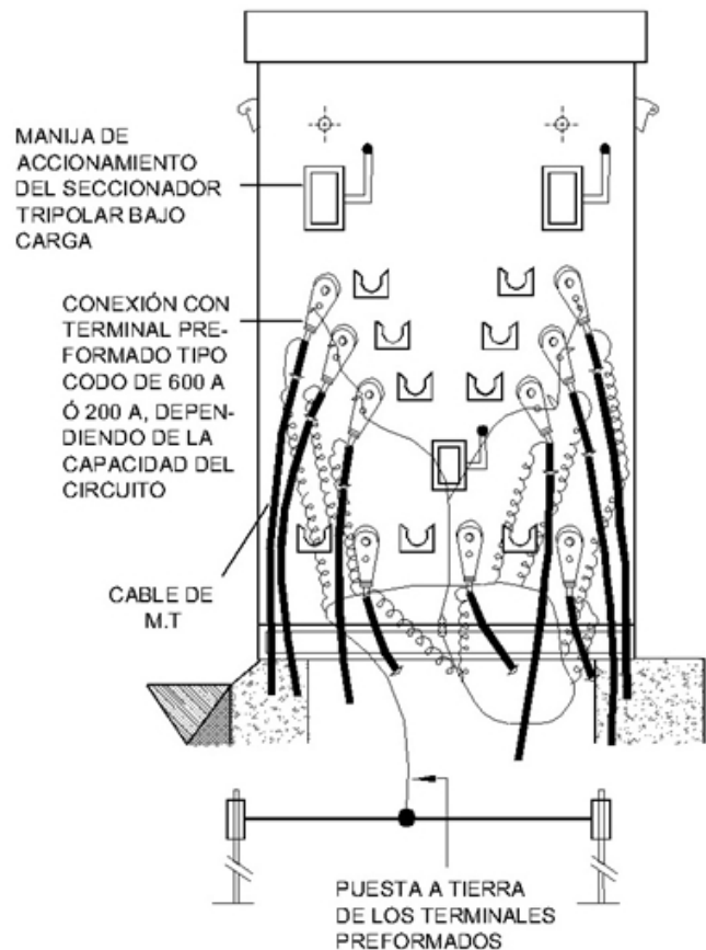
CAJAS DE MANIOBRA TIPO PEDESTAL
