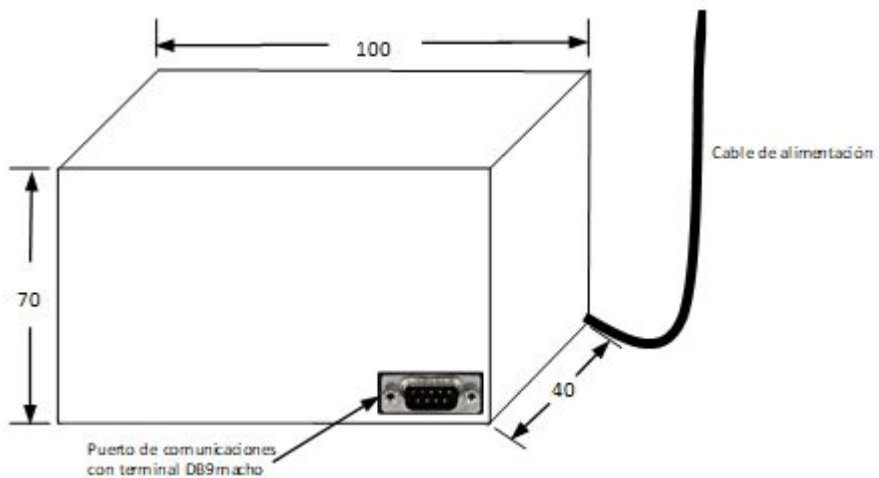
FIGURA 2. DIMENSIONES MODULO EMISOR
