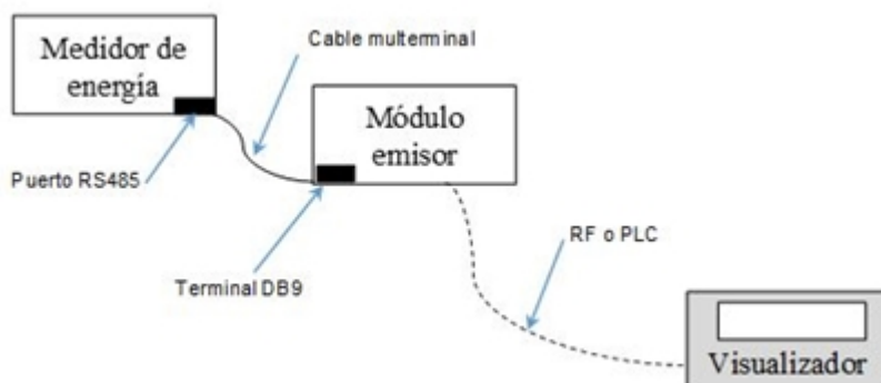
FIGURA 1. ESQUEMA REPETIDOR
