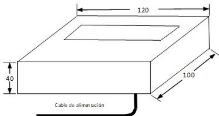
FIGURA 3. DIMENSIONES MODULO VISUALIZADOR
