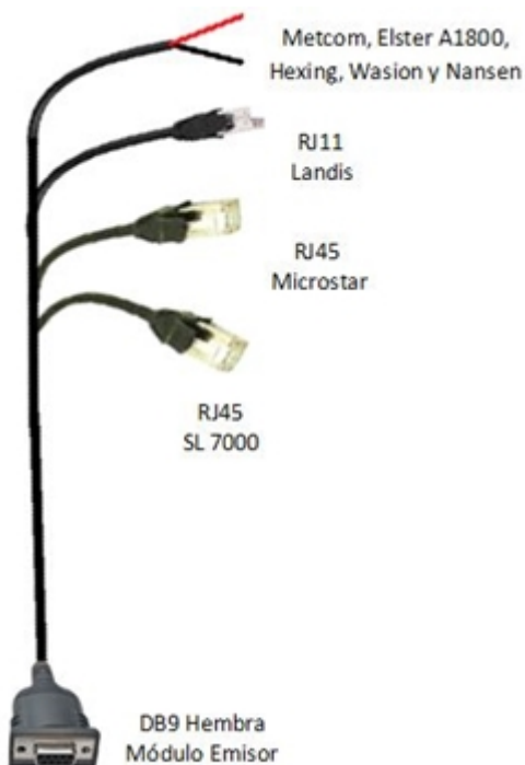
FIGURA 4. CABLE DE COMUNICACIONES
