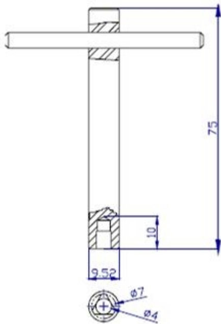
FIGURA 3. LLAVE PARA PERNO DE CABEZA TRIANGULAR
