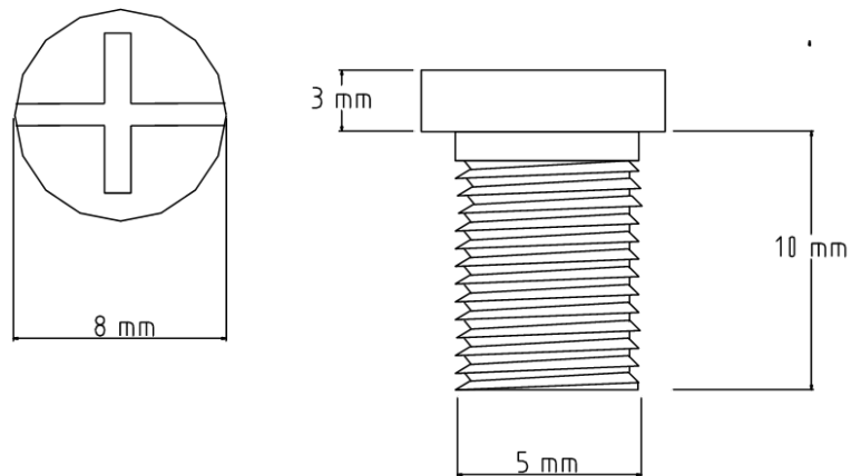
FIGURA 4. PERNO DEL SISTEMA DE SEGURIDAD
