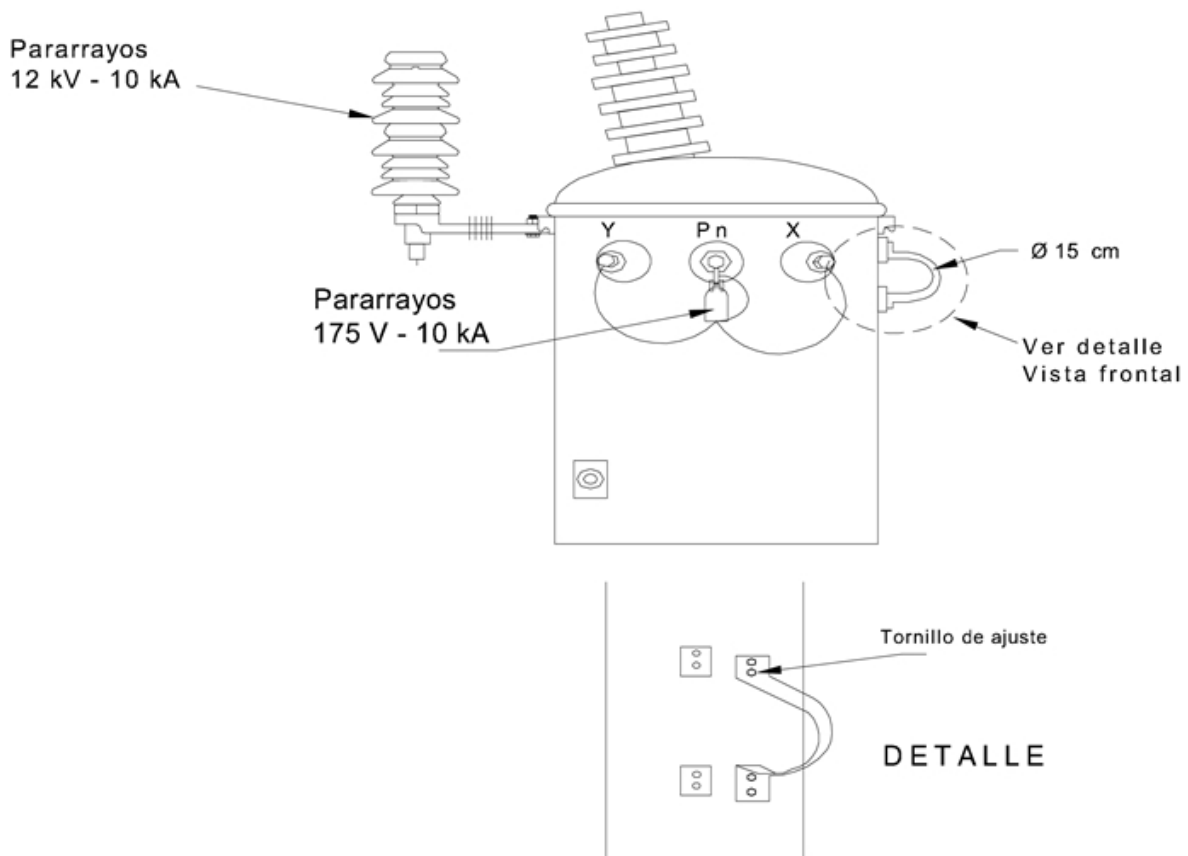
FIG.1. DISPOSITIVO DE TRANSPORTE INTERCAMBIABLE
