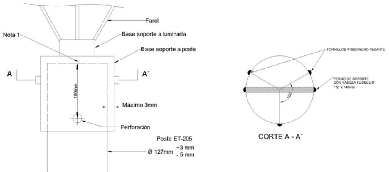
Figura No 1 Sistema de montaje de la base de la luminaria al poste
