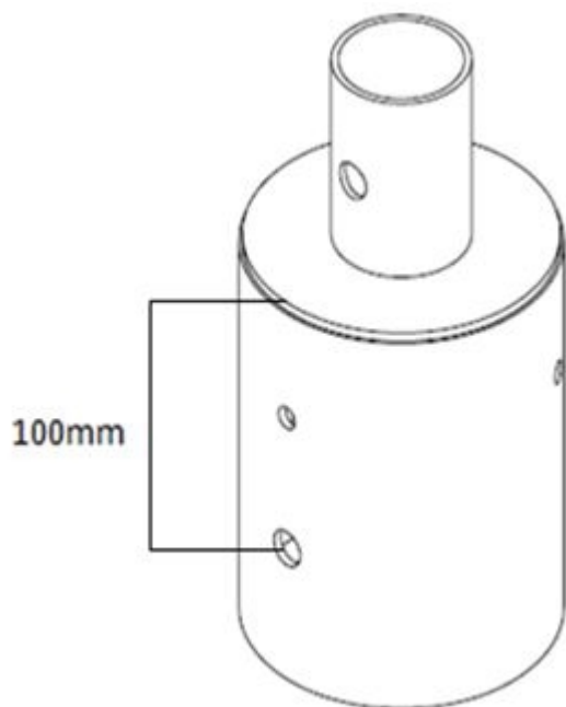
Figura No. 2 Vista isométrica base a poste
