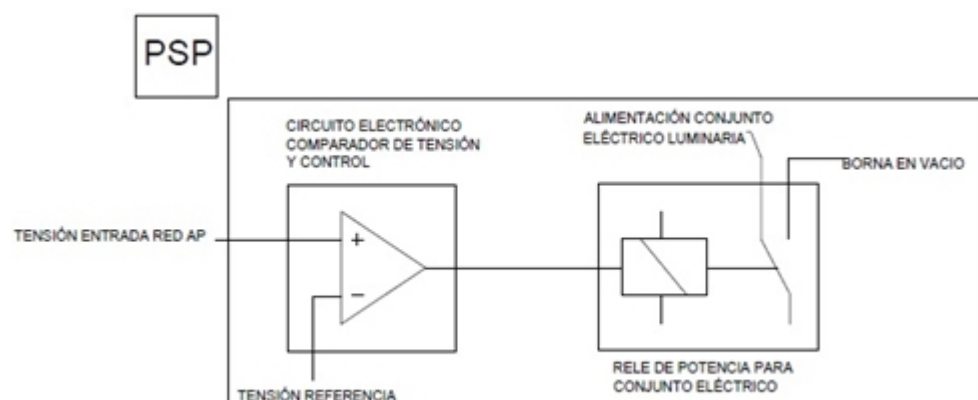
Figura No. 2 Diagrama electrónico del PSP
