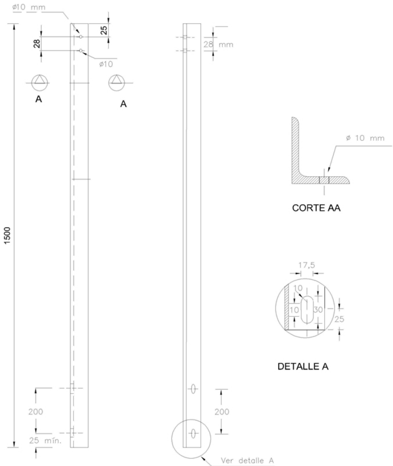
FIGURA 1 BAYONETAS PARA ALINEAMIENTOS
