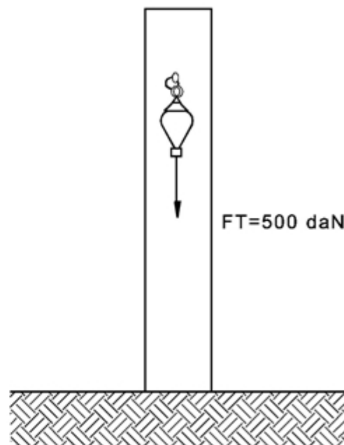
FIG. 4 ENSAYO DE TRACCIÓN
