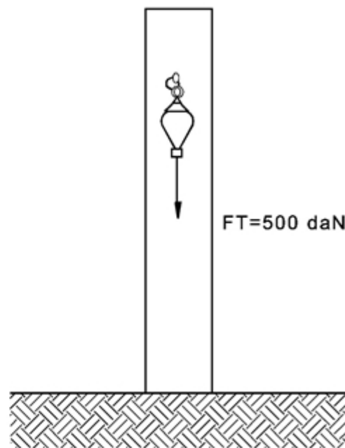
FIG. 4 ENSAYO DE TRACCIÓN
