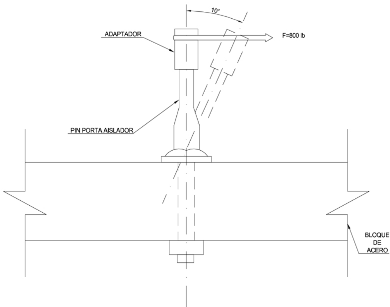
FIGURA 2: ENSAYO DE TRACCIÓN Y FLEXIÓN
