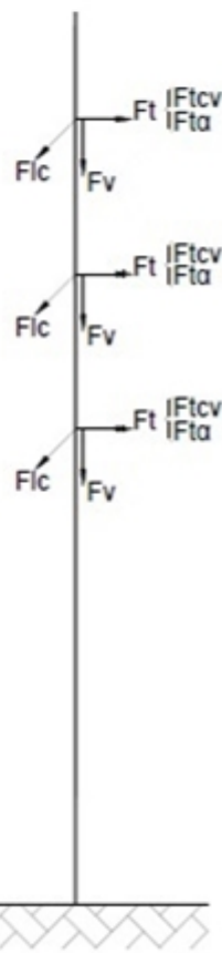
DIAGRAMA DE CARGAS EN ALZADO
