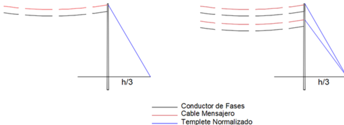
Figura 3. Disposición para la instalación de templetes
