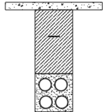
CUATRO DUCTOS DE Ø 6" CS 217-1
