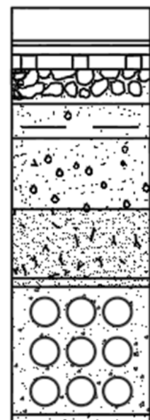
CRUCE PASO NIVEL LINEAS FERREAS A CONSTRUIR. DETALLES DUCTOS, 9 DUCTOS 6" CS 222-1
