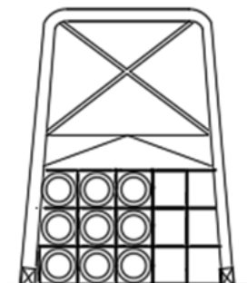
DUCTOS GALVANIZADOS SOBRE ESTRUCTURA CS 218-1
