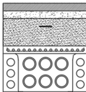
DETALLE GENERAL DE DUCTOS, ZANJA Y RELLENOS PARA 6 DUCTOS DE Ø 6" CON SARDINEL PREFABRICADO, APLICABLE SEGÚN DISEÑO JUSTIFICADO CS 221-2
