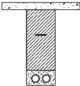
DO S DUCTOS DE Ø 4" CS 208-1
