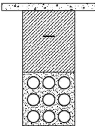
NUEVE DUCTOS DE Ø 6" CS 213-2
