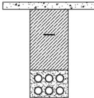
SEIS DUCTOS DE Ø 4" CS 210-1
