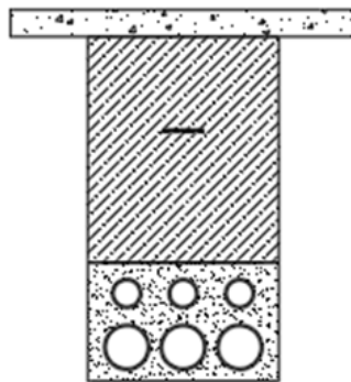
TRES DUCTOS DE Ø 4" Y TRES DUCTOS DE Ø 6" CS 214-1
