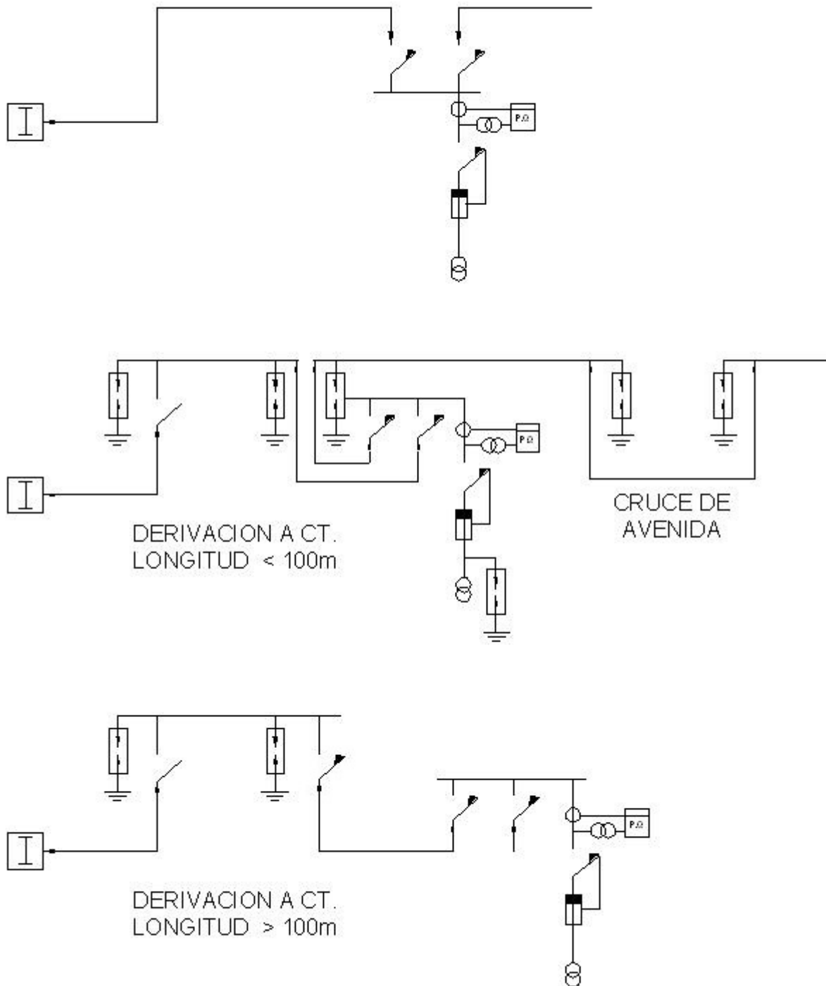
FIG. 3.1 ESQUEMA BÁSICO PRIMARIO. C
