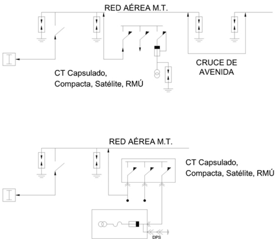
FIG 3.1 ESQUEMA BÁSICO PRIMARIO. B
