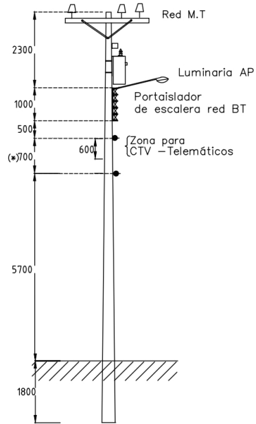
POSTE DE 12m CON TRANSFORMADOR
