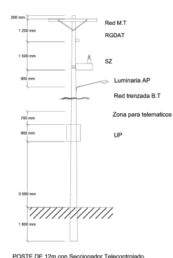
POSTE DE 12m con Seccionador Telecontrolado, luminaria y red trenzada BT
