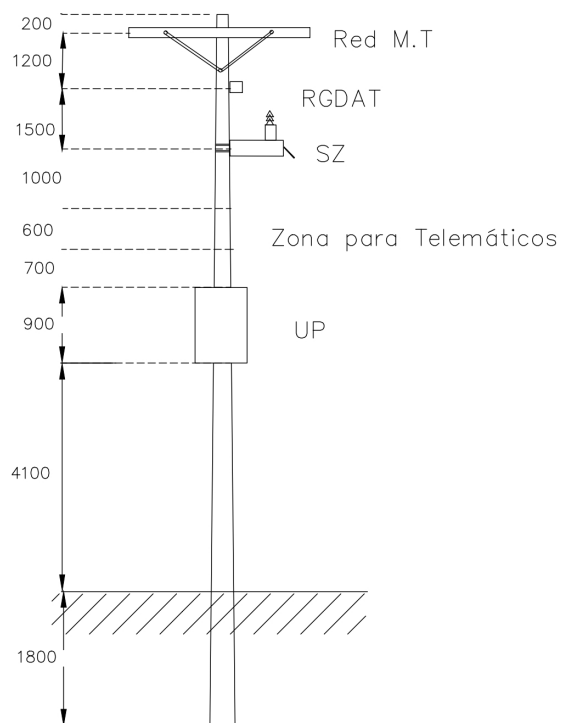
Poste de 12 m con Seccionador Telecontrolado
