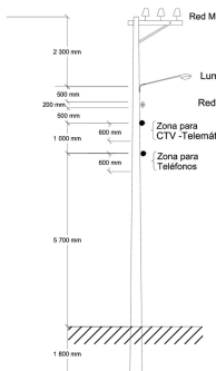
POSTE DE 12 m RED DE M.T. y B.T
