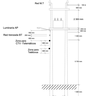
POSTE DE 12 m ESTRUCTURA TIPO H
