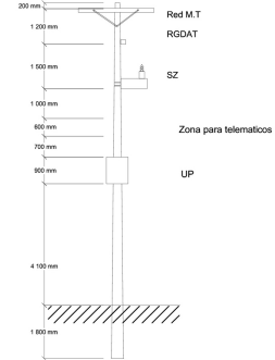
POSTE DE 12m con Seccionador Telecontrolado
