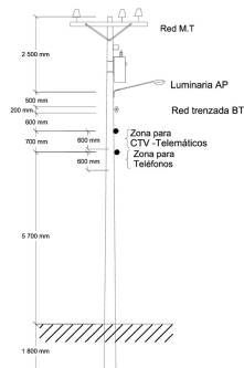
POSTE DE 12m CON TRANSFORMADOR
