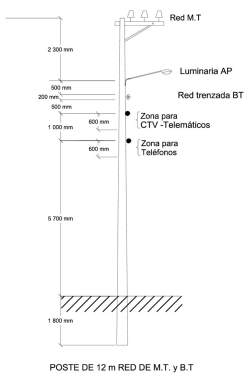
POSTE DE 12 m RED DE M.T. y B.T
