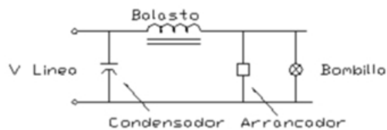
Disposición Balasto reactor para luz de sodio
