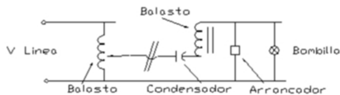
Disposición Balasto CWA (Autoregulado) para luz de sodio
