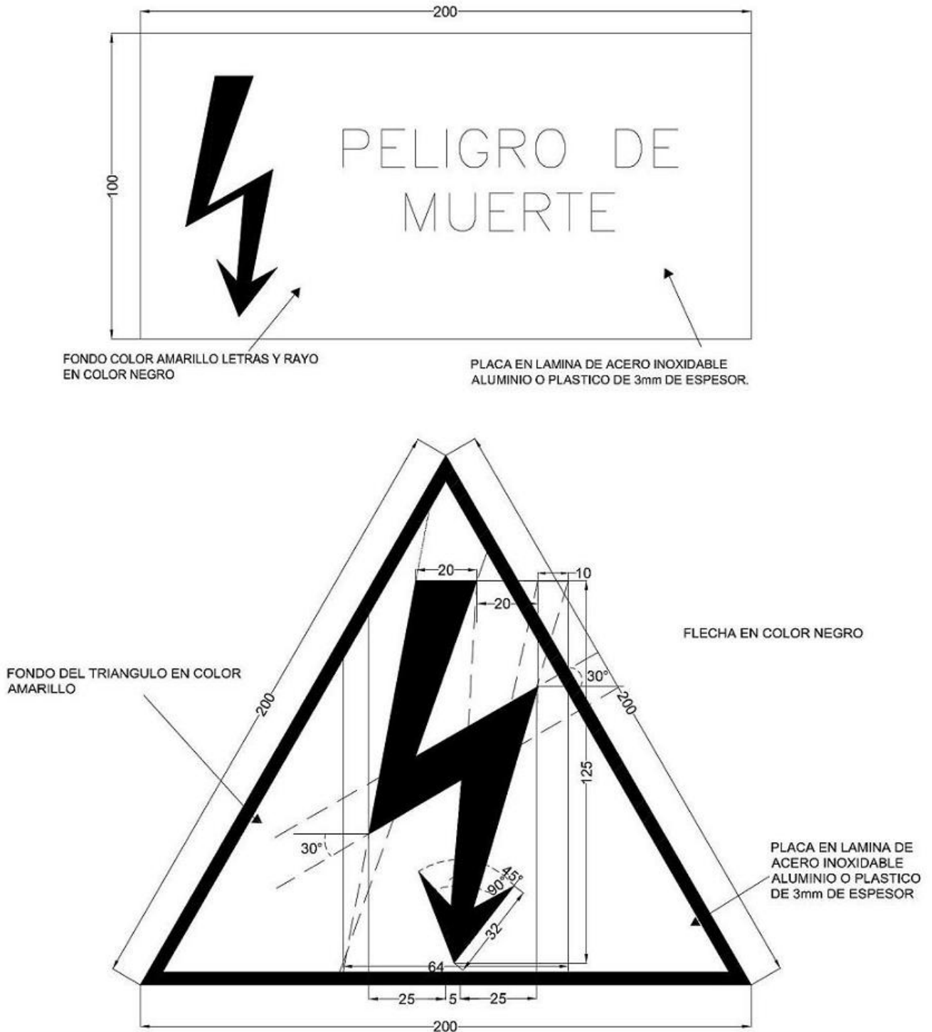
FIGURA 1 SEÑAL PREVENTIVA.
