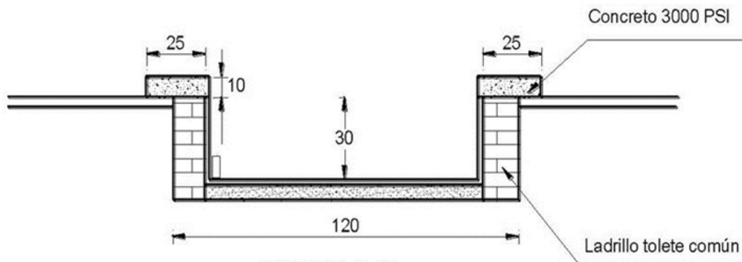
CORTE A-A'
