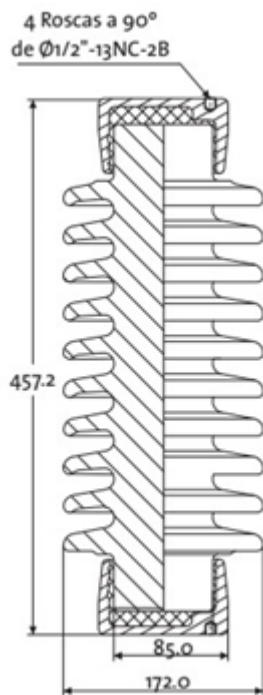
Figura 3. Dimensiones aislador soporte 36 kV
