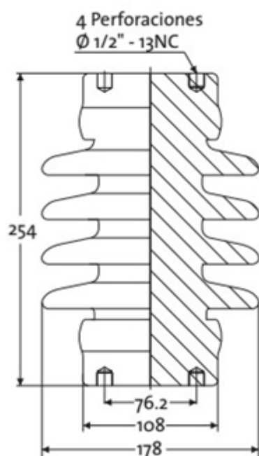
Figura 2. Dimensiones aislador soporte 17,5 kV
