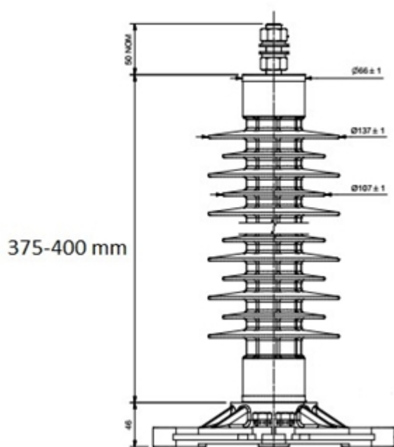
Figura 1. Dimensiones descargadores de sobretensión 12 y 30 kV
